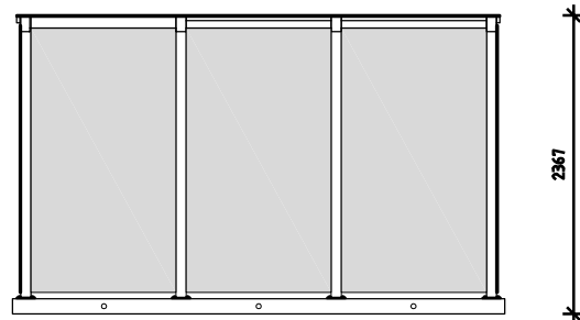
Vorderansicht
